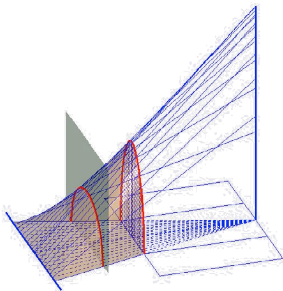
Imaxe 26: Tetraedroide
