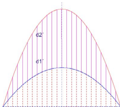
Imaxe 15: Obtención das xeratrices do cilindroide. Alzado
