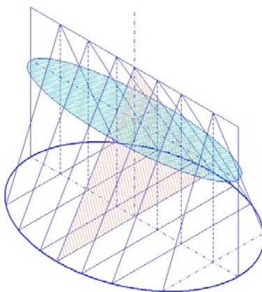
Imaxe 9: Conoide
